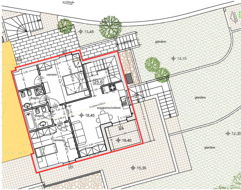
PIANO SOTTOTETTO
